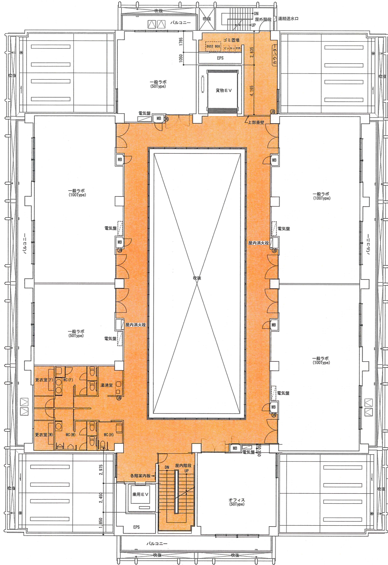
1号館 4階平面図
