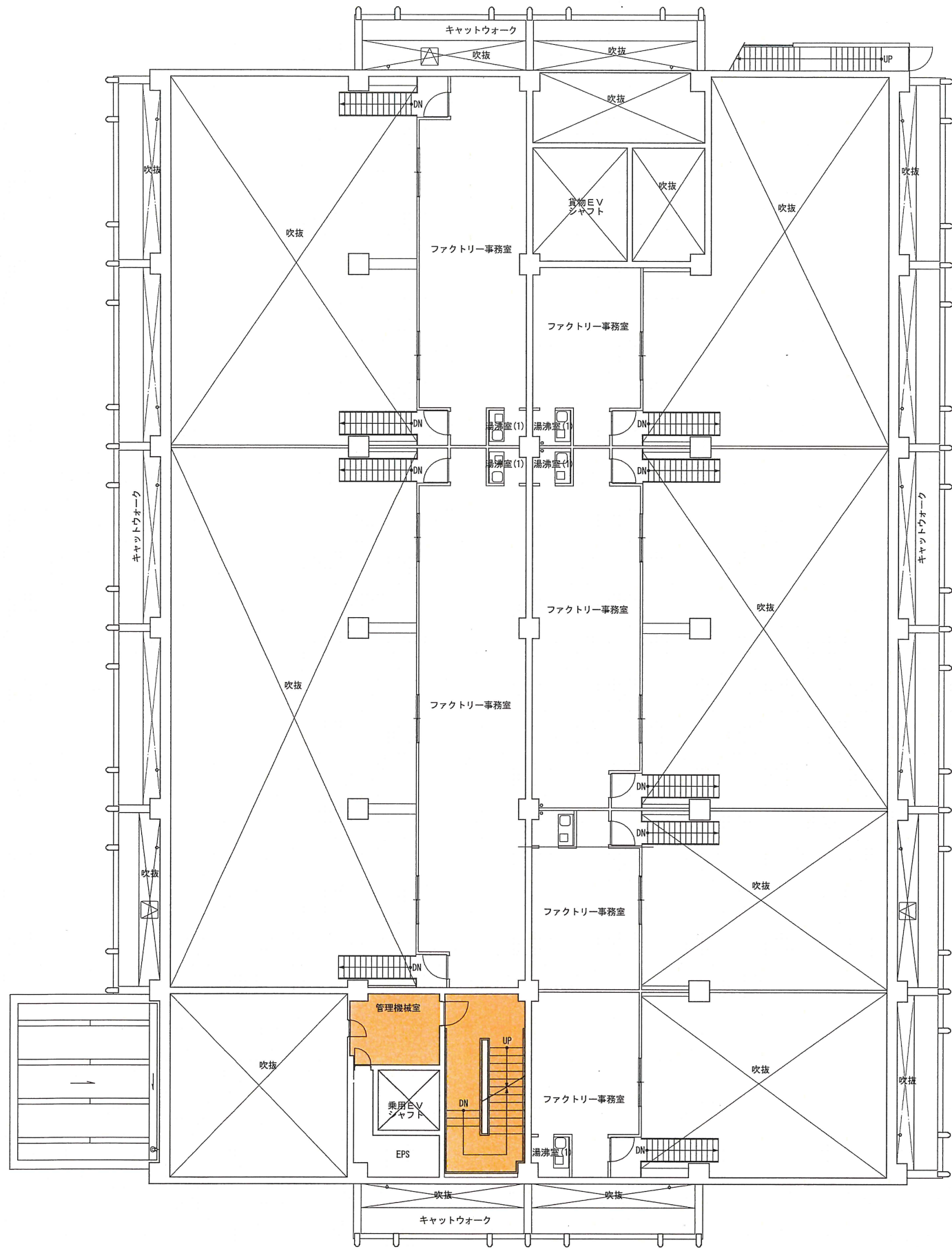
1号館 中2階平面図
