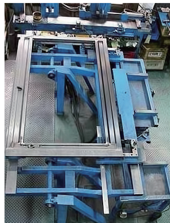
溶接治具
