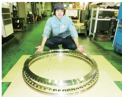
半導体ウェハのポリシング機に超大型スラスト玉軸受
