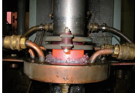
ロールの高周波焼入れ
