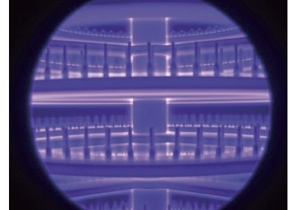
ピストンロッドのプラズマ窒化
