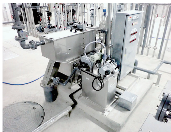
TONPARA 污泥濃縮機
