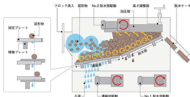
SPATON テクノロジー構造
