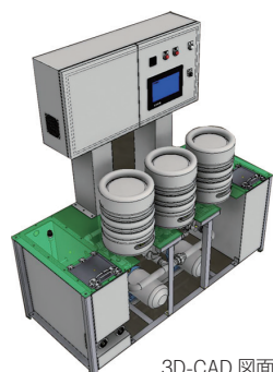
3D-CAD 図面
