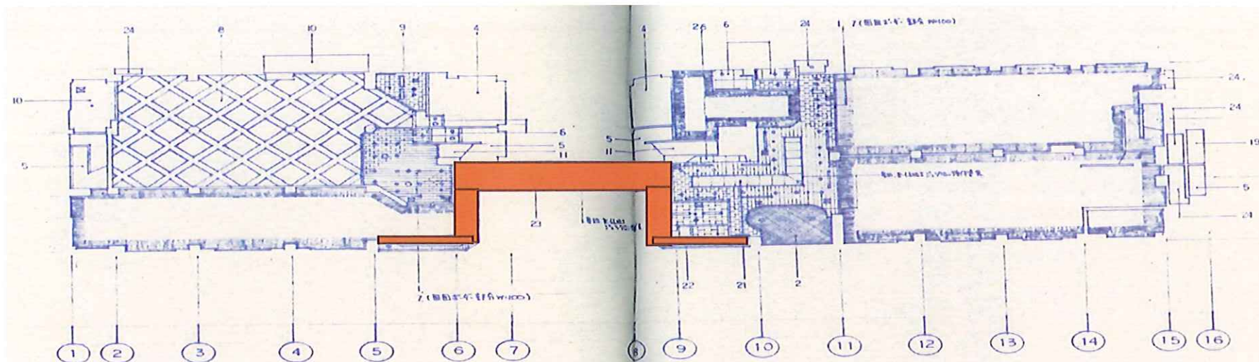
1 階天井伏図
