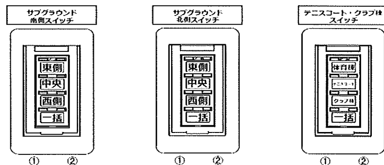
メイン棟2階事務所 スイッチ外観図
