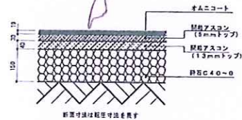
砂入り人工芝舗装断面図
