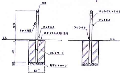
テニスネットポスト詳細図
