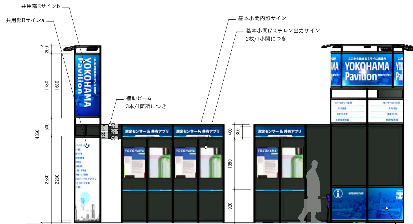
01 立面
