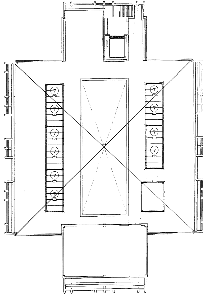
(LVP-1) 6階平面図 S=1/150
