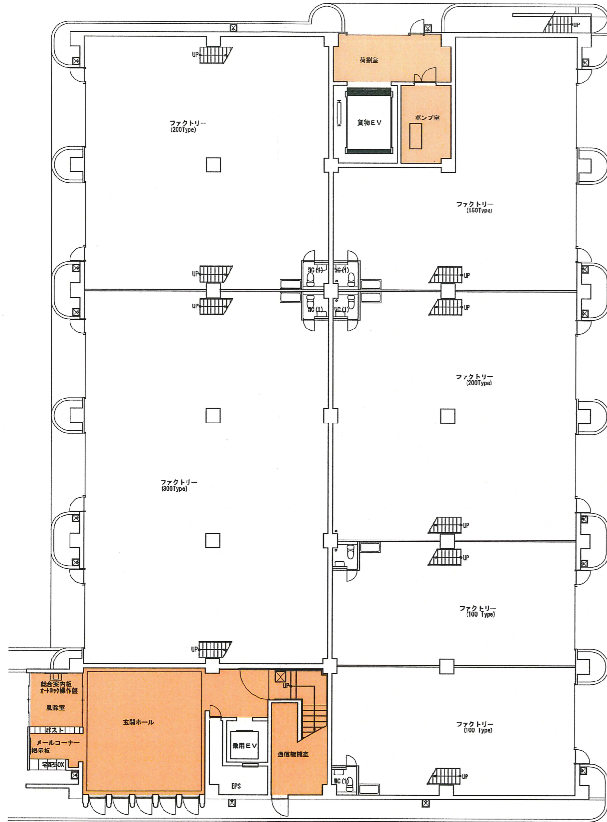
1号館 1階平面図
