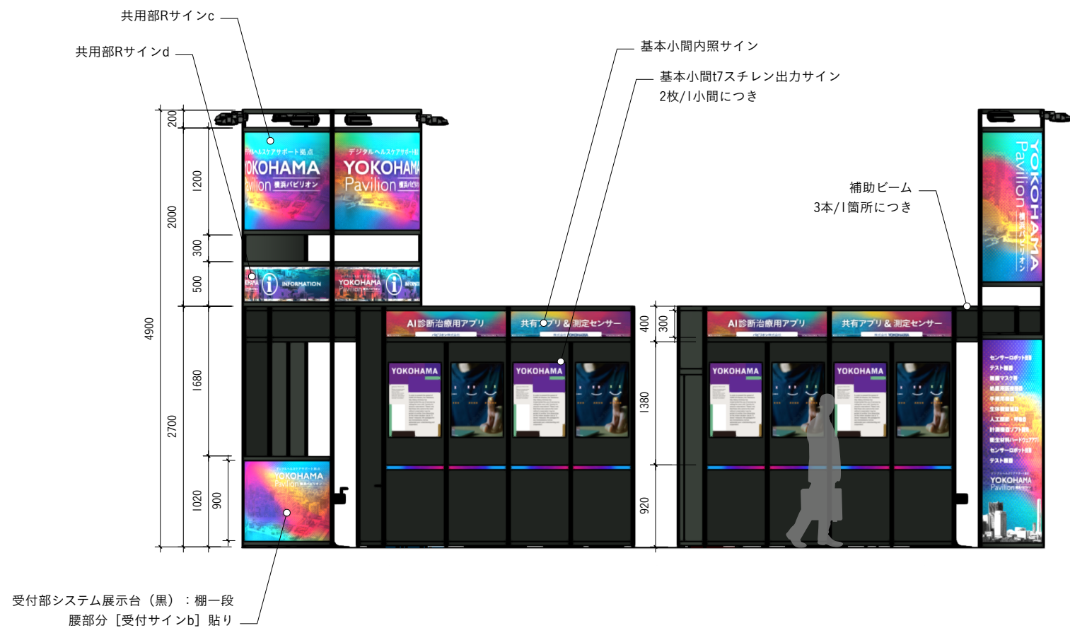
01 立面
