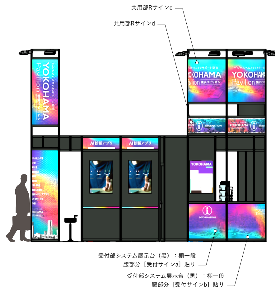
04 立面
