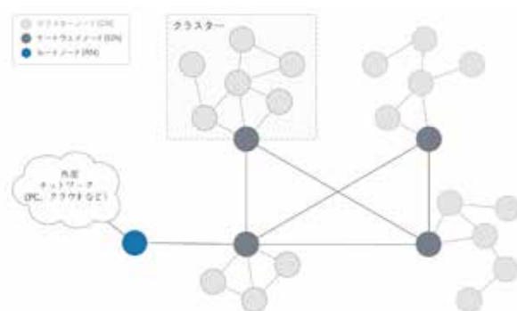
Fig2. 独自無線メッシュネットワーク (A-net)
